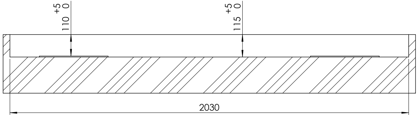
SCHNITT A-A
