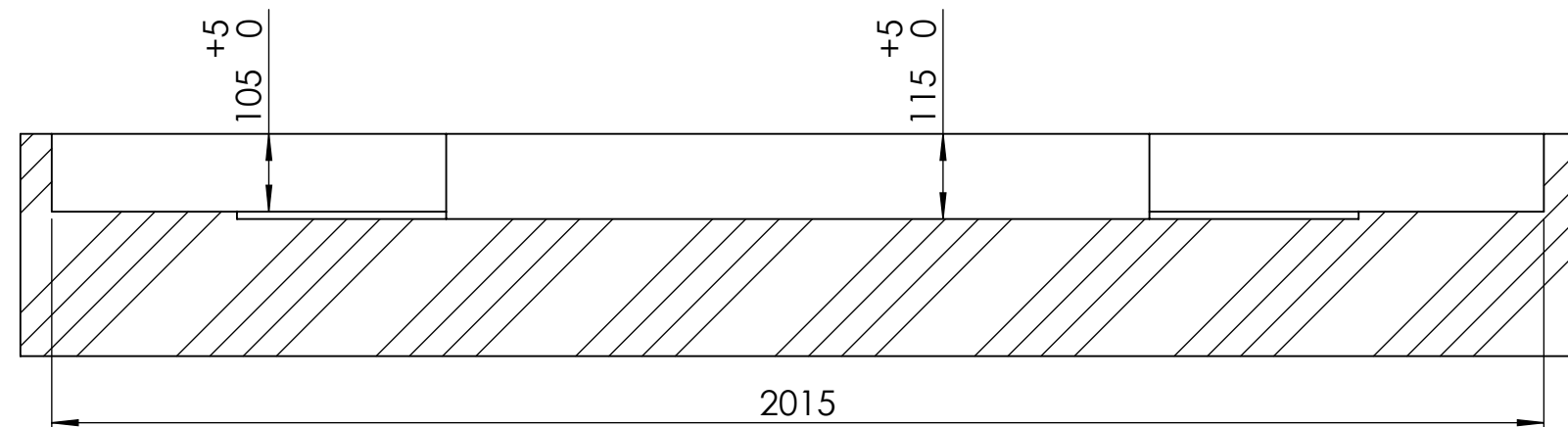
SCHNITT A-A
