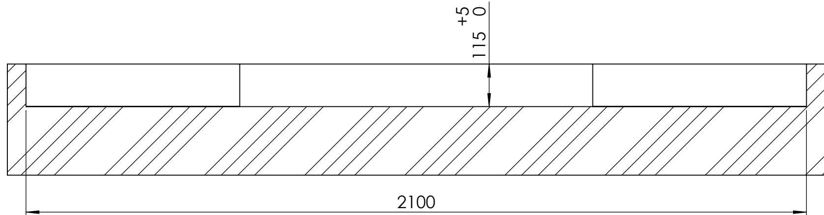
SCHNITT A-A
