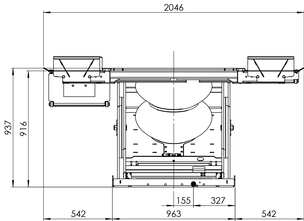
Bodenverschraubung/Bottom screwing
