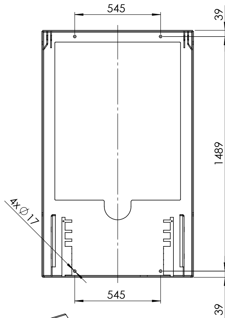
Bodenverschraubung/Bottom screwing
