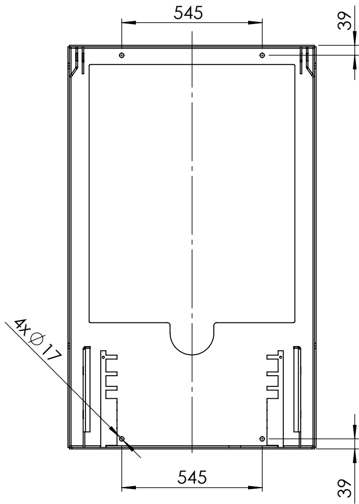
Bodenverschraubung/Bottom screwing
