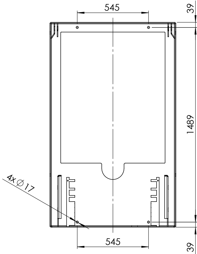
Bodenverschraubung/Bottom screwing
