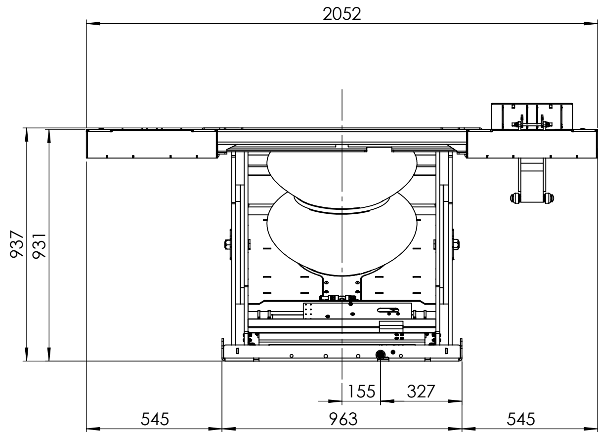
Bodenverschraubung/Bottom screwing
