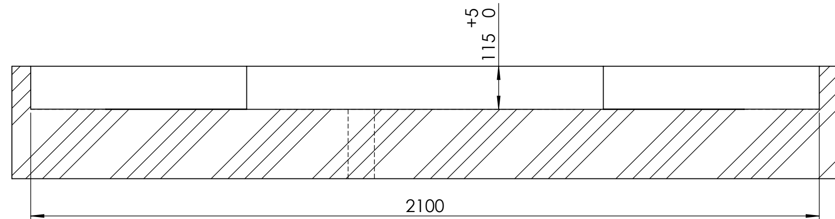
SCHNITT A-A
