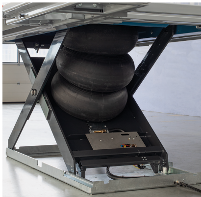
Das Herzstück jeder pneumatischen Hebebühne – der Luftbalg
