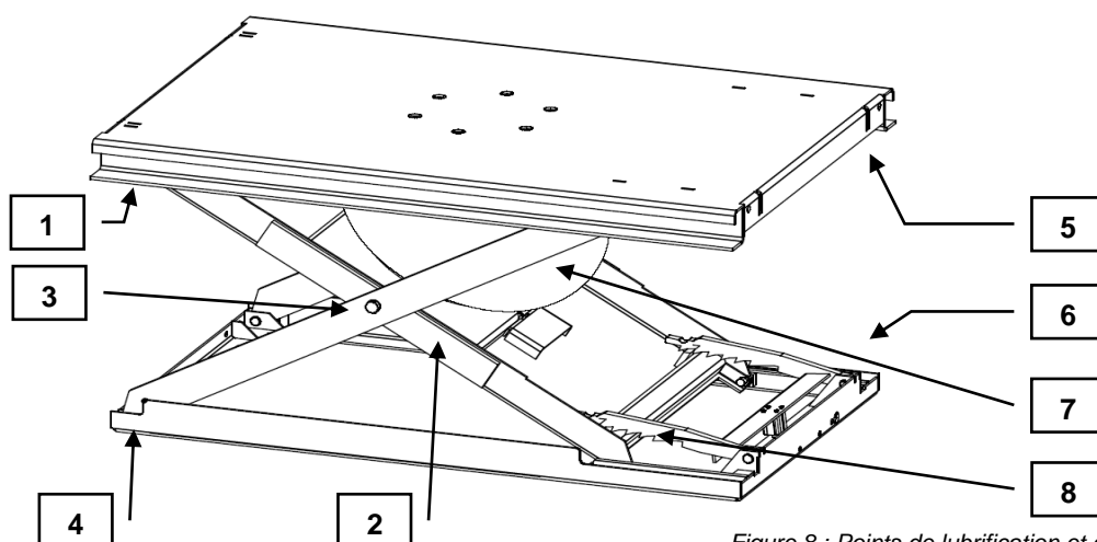
Figure 8 : Points de lubrification et de contrôle
