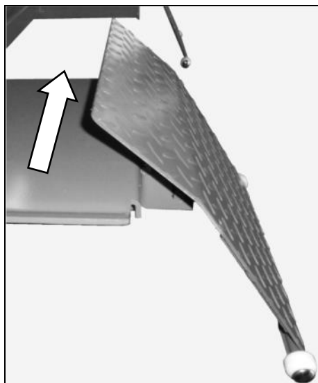
Image : Table élévatrice en position haute avec rampe de montée installée
