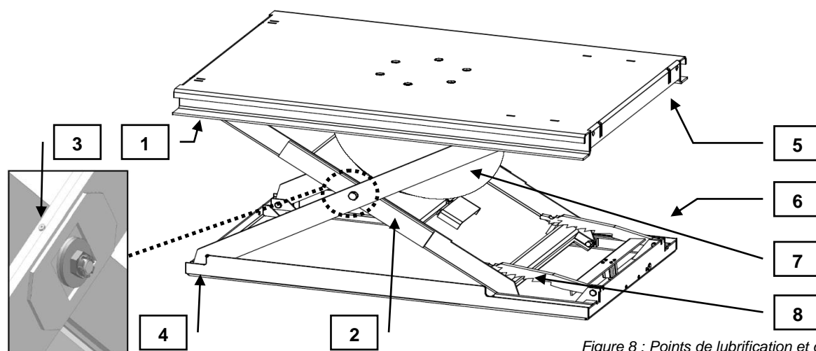
Figure 8 : Points de lubrification et de contrôle
