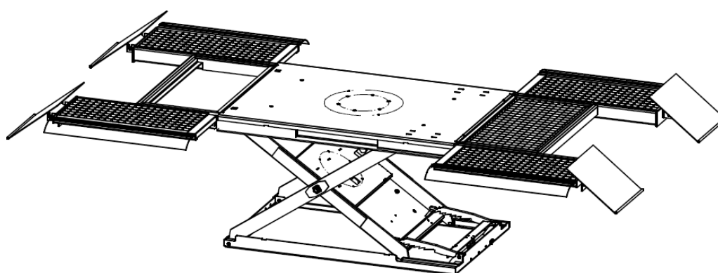
Figure 2 : Produit HLS1200-14/-16
