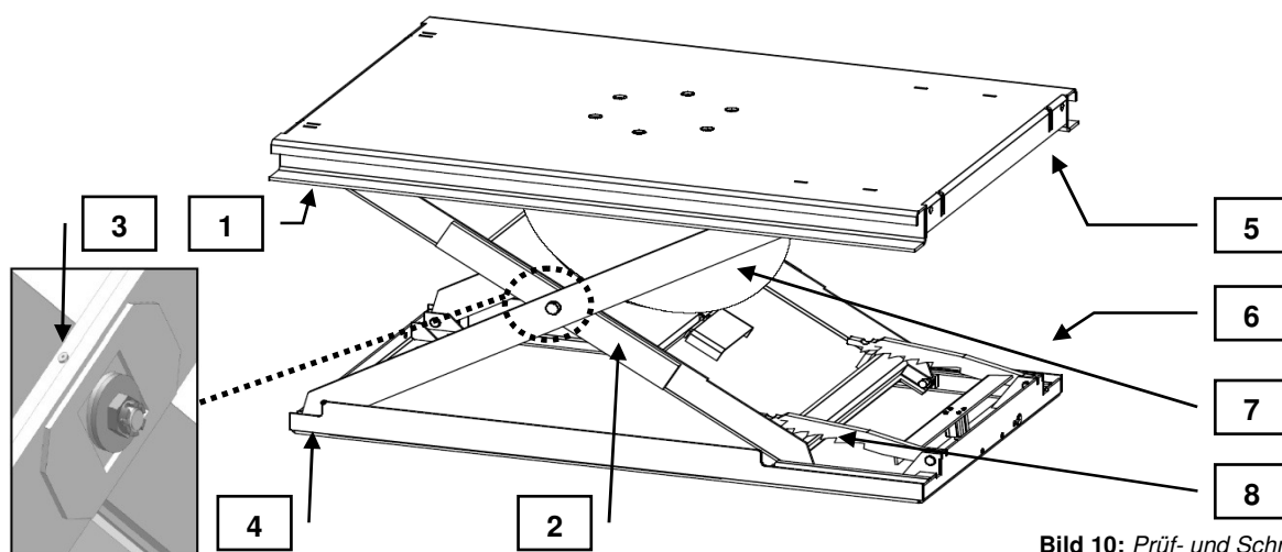
Bild 10: Prüf- und Schmierpunkte
