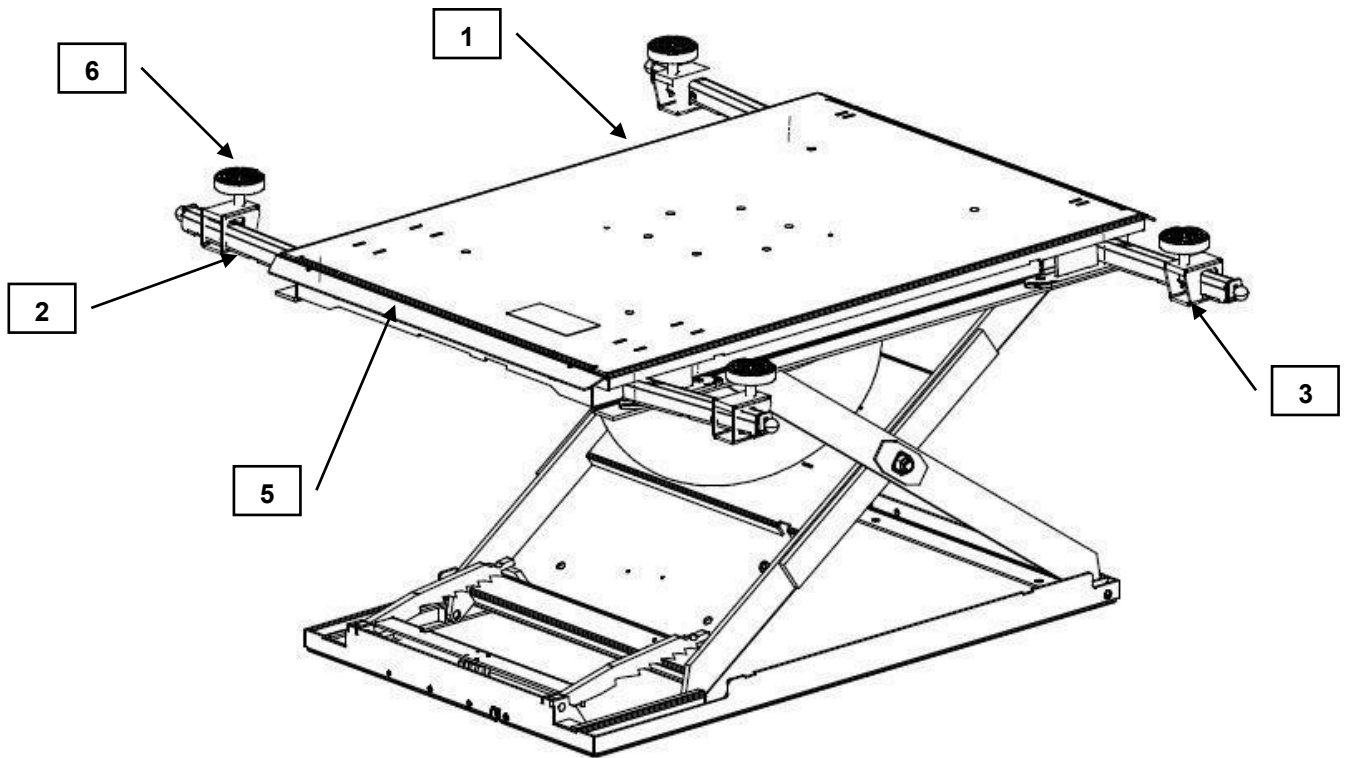
Bild 9: HM1100-01
