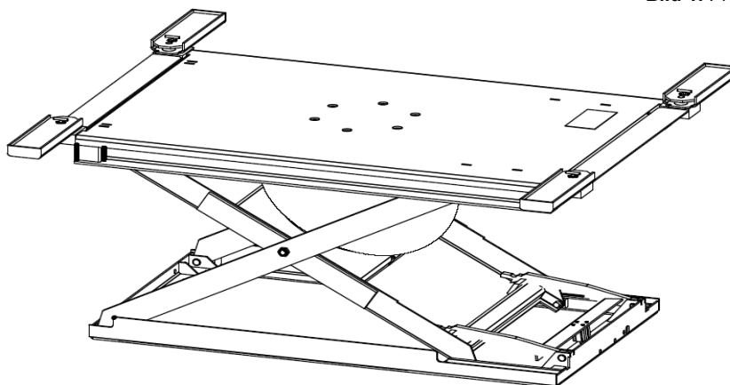
Bild 1: Produkt HM1100-01
