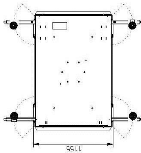
Bild 12: Maßblatt HM1100-01
