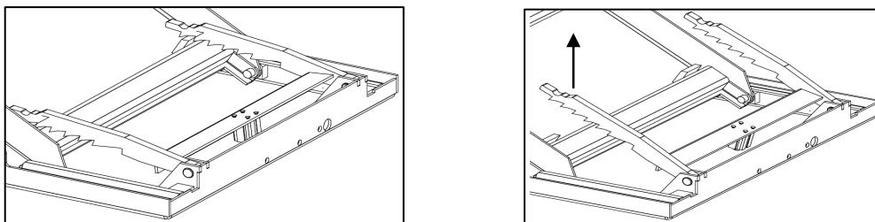
Bild 3 /4: Fallsicherung eingerastet / Fallsicherung angehoben beim Senkvorgang
