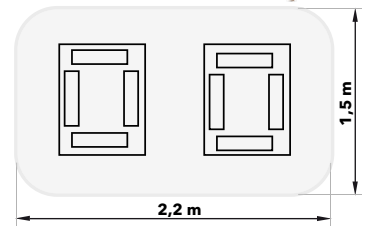
IRT 4-20 PCAUTO Deux cassettes à une distance de 600 mm sur du métal de feuille noire.
